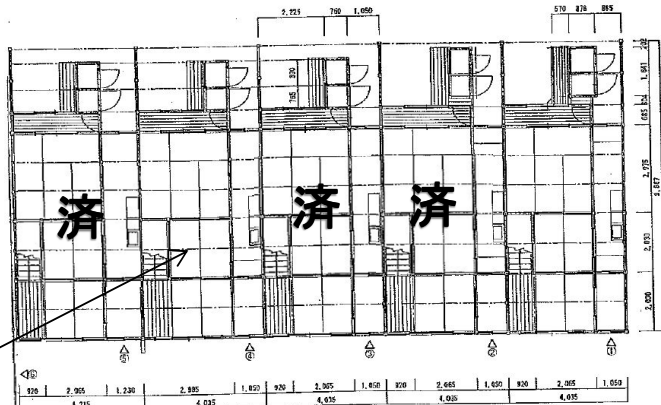
1階平面図
